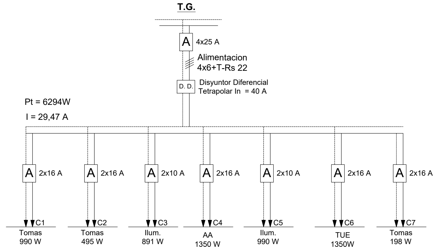
ESQUEMA DE TABLEROS
