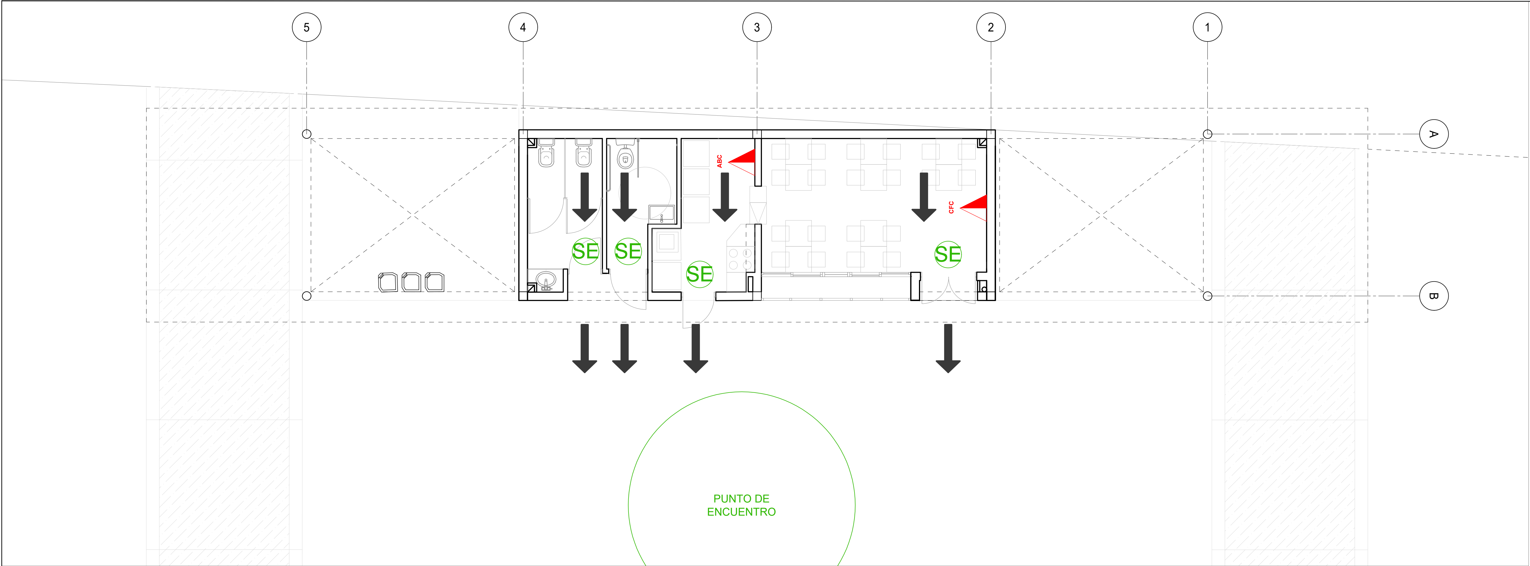
Plaza Timbo PLANTA DE SERVICIO CONTRA INCENDIOS
